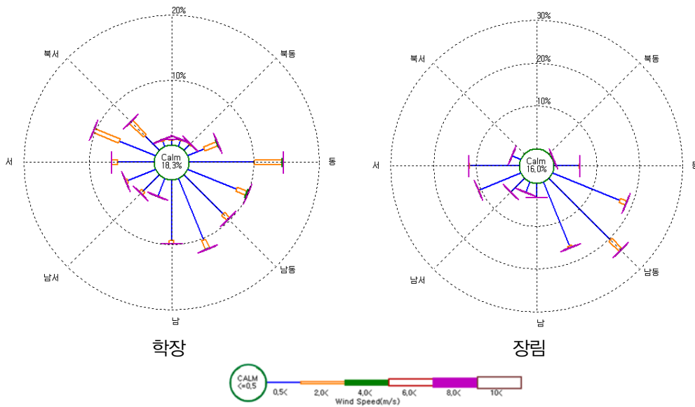
그림 7. 지점별 풍배도
