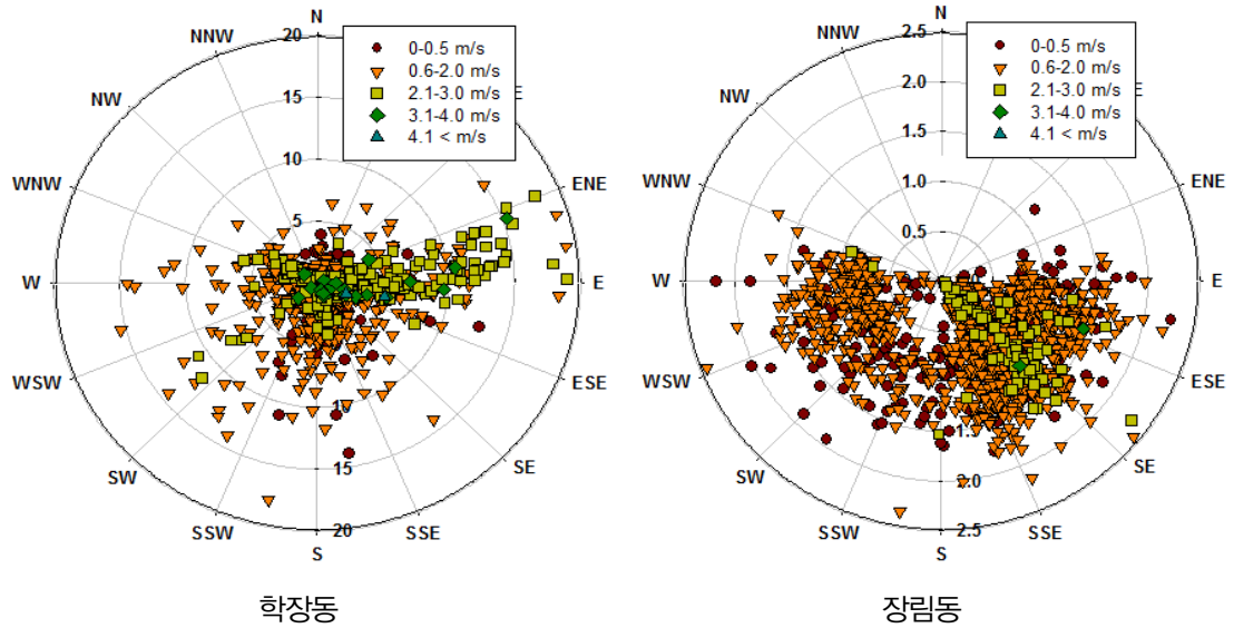
그림 6. 벤젠 오염장미
