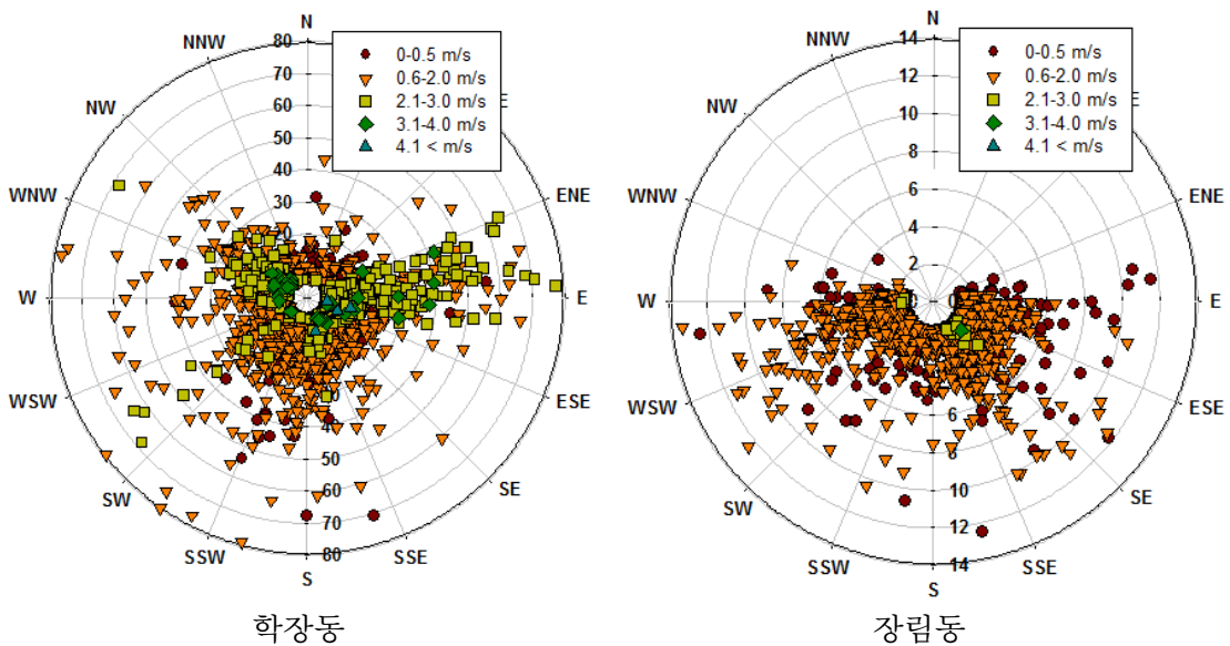
그림 6. 톨루엔 오염장미
