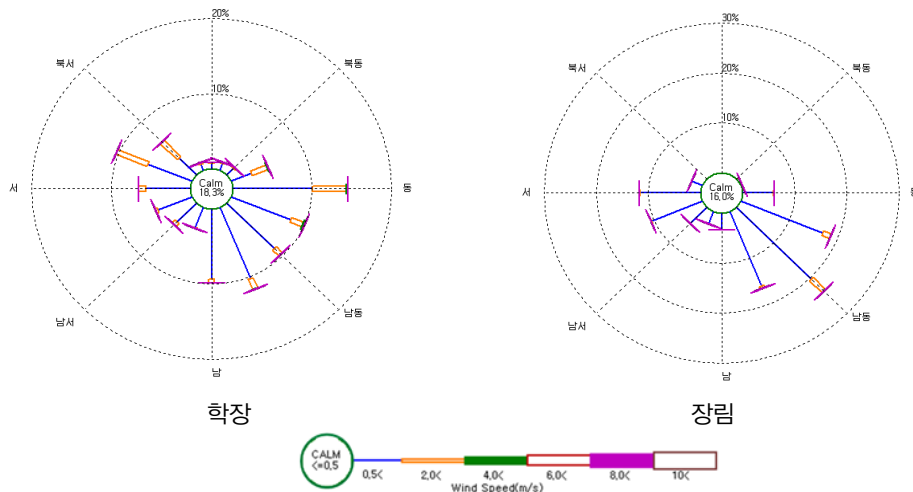
그림 2. 2016년 풍배도
