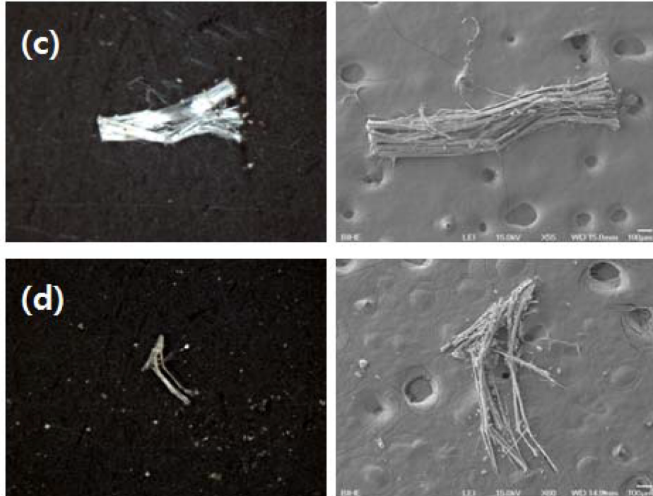
그림 3. 퇴적먼지 중 석면 (a)범천동(노후슬레이트주거지역), (b)철마면(슬레이트축사), (c)남향동(수리조선소주변), (d)엄궁동(폐기물처리시설주변)
