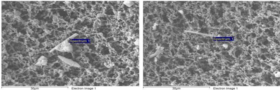
그림 2. 대기 중 무기섬유입자 (a)좌천동(노후슬레이트주거지역), (b)다대동(수리조선소주변)
